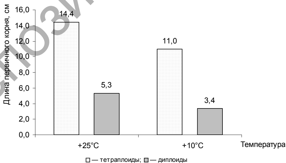
Рисунок 1. — Длина первичного корня гречихи в зависимости от пloidности сорта
