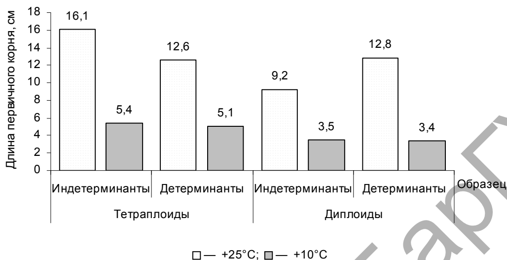
Рисунок 2. — Длина первичного корня гречихи в зависимости от морфотипа сорта и его плоидности
