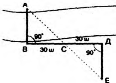
Рис. 11 – Определение ширины реки методом шагов
