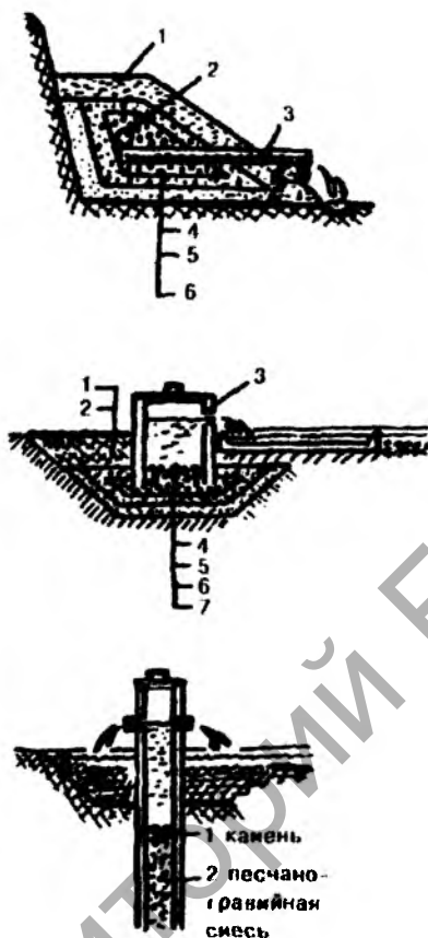
Рис.12 — Устройство водоприемника на роднике: 1 - пористый грунт; 2 - дренажная труба; 3 - отводящая труба; 4 - щебень; 5 - песчано-гравийная смесь; 6 - песок; 1 - камень; 2 - глина; 3 - труба; 4 - камень; 5 - щебень; 6 - песчано-гравийная смесь; 7 - песок.
