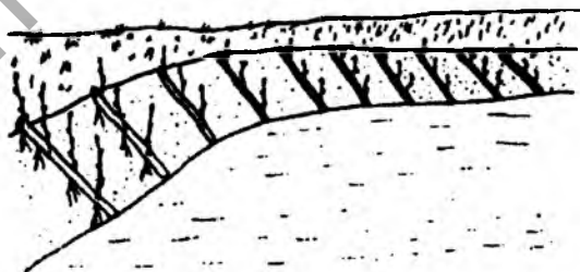
Рис. 15 — Укрепление берегов речки при помощи наклонно прикопанных кольев ивы
