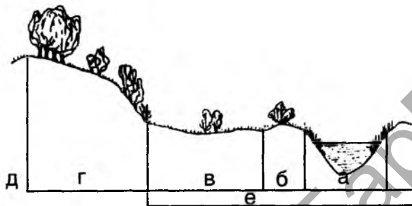
Рис. 2 — Строение речной долины: а – русло, б – предрусловый вал, в – пойма, г – пойменная терраса, д – водораздел, е – речная долина.
