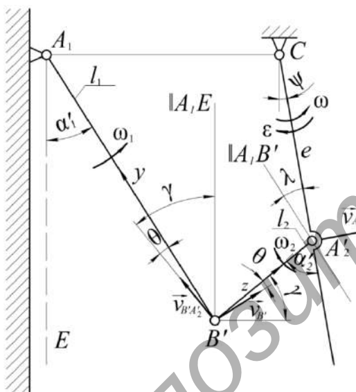
Рысунак 14 – Ілюстрацыя да вызначэння скорасцей пунктаў і звенняў
