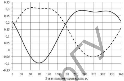
Рысунк 28 – Графік змянення кампаненты X_{A_1}^d : сцэпная лінія – для левага палова рабочай камеры, пункцірная – для правага
