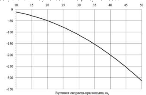
Рысунк 30 – Графік змянення тангенцыяльнай дынамічнай сілы R_{A_2}^{nt} ўзаемадзеяння левага рабочага органа з каромыслам (крайняе левае становішча каромысла – \psi = 8,19^\circ )
