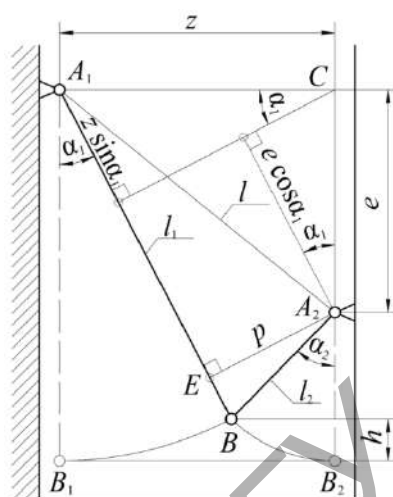
Рисунок 3 – Ілюстрація да вызначэння геаметрычных суадносін пры вертыкальным становішчы каромысла
