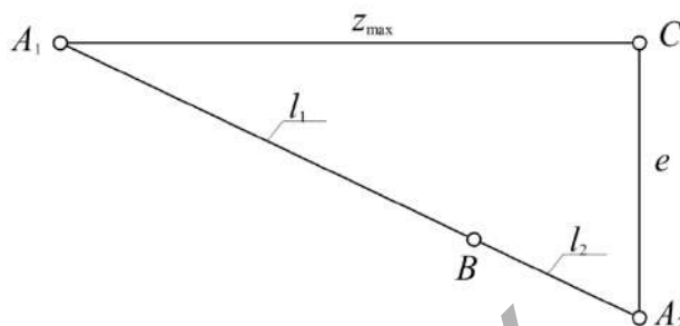
Рысунк 13 – Ілюстрацыя да вызначэння велічыні z_{\text{max}}
