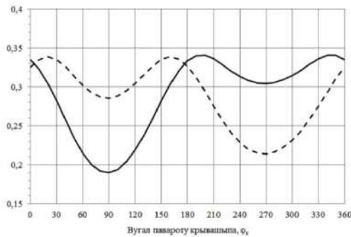
Рысунк 25 – Графік змянення нармальнай кампаненты R_{A_2}^{nn} сілы ўзаемадзеяння рабочых органаў з каромыслам: сцэпная лінія – для левага палова рабочай камеры, пункцірная – для правага
