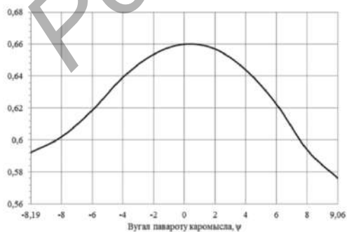
Рысунк 27 – Графік змянення раўнадзейнай \bar{R}_{A_2}^d сілы ўзаемадзеяння двух рабочых органаў з каромыслам
