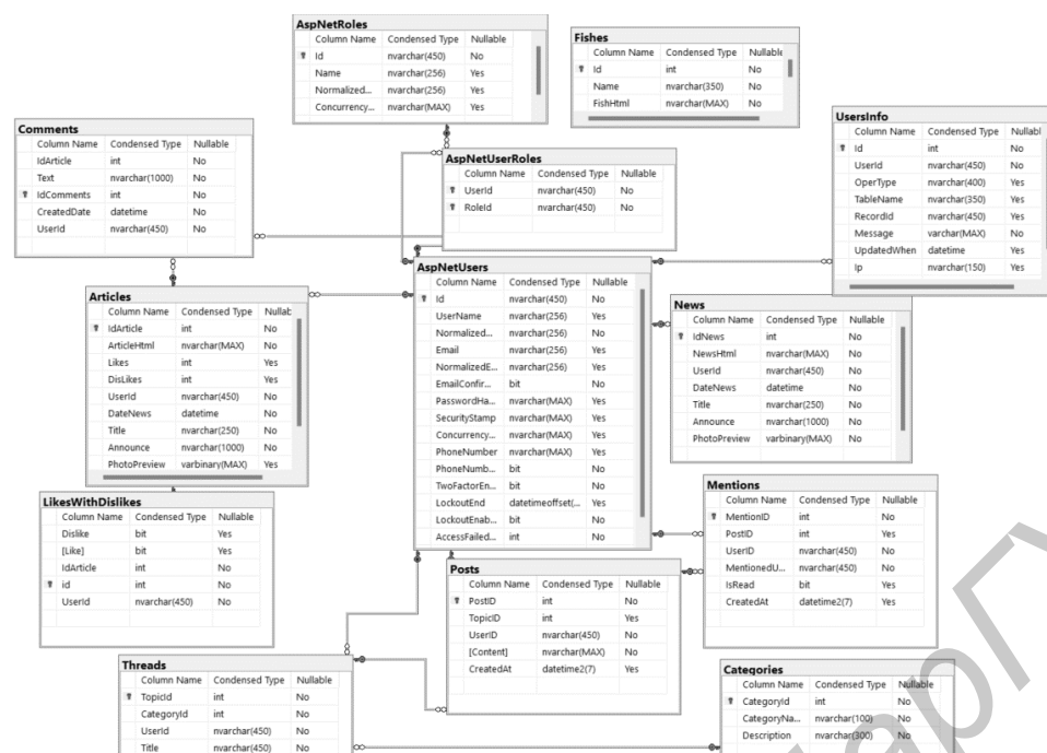
Рисунок 3 — Физическая модель базы данных веб-сайта для рыболовов
