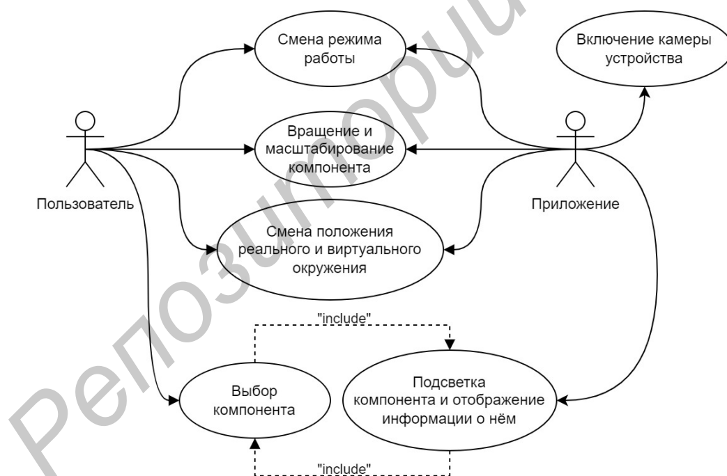
Рисунок 1 — Диаграмма вариантов использования проектируемого приложения
