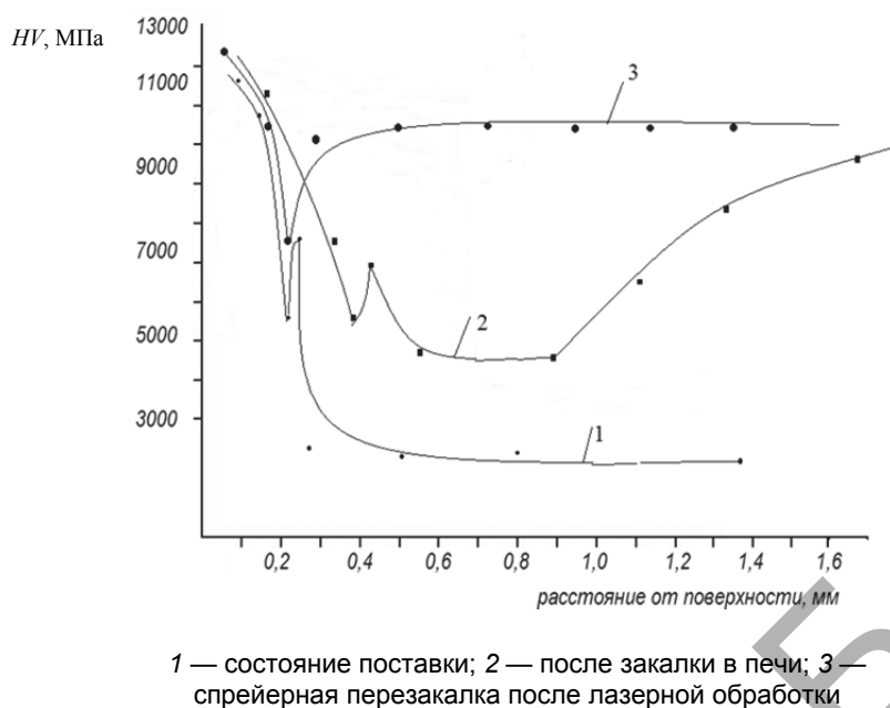
Рисунок 1. — Изменение микротвердости при лазерном модифицировании стали 9ХФ при различной исходной структуре подслоя
