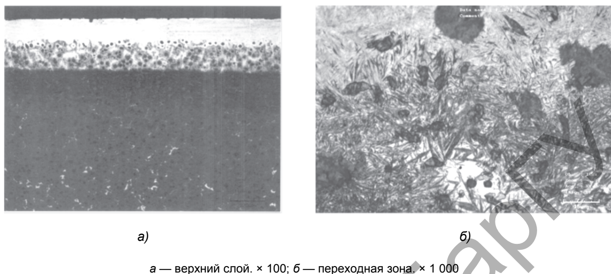
Рисунок 2. — Микроструктура зоны лазерного упрочнения бейнитного чугуна
