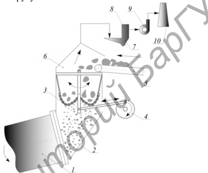
Рис. 1. Набор оборудования для измельчения и сушки мела в технологии производства извести. 1 — вращающаяся печь; 2 — пыльная камера; 3 — цепной агрегат; 4 — привод цепного агрегата; 5 — ленточный конвейер; 6 — газоход; 7 — пылесборник; 8 — электрофильтр; 9 — дымосос; 10 — труба
