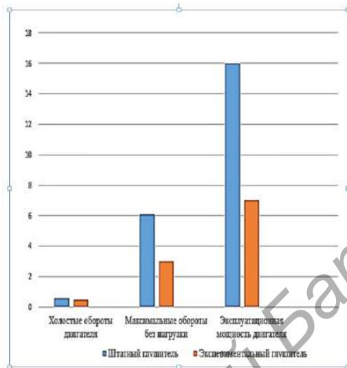
Рис. 2. Сопrotивление выхлопным газам, кПа
