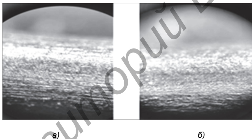
Рисунок 4. — Сравнительные испытания необработанных (а) и предварительно обработанных (б) образцов на питтинговую коррозию
