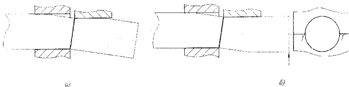
а — обычная резка, б — качественная резка с поддержкой отрезаемой заготовки
