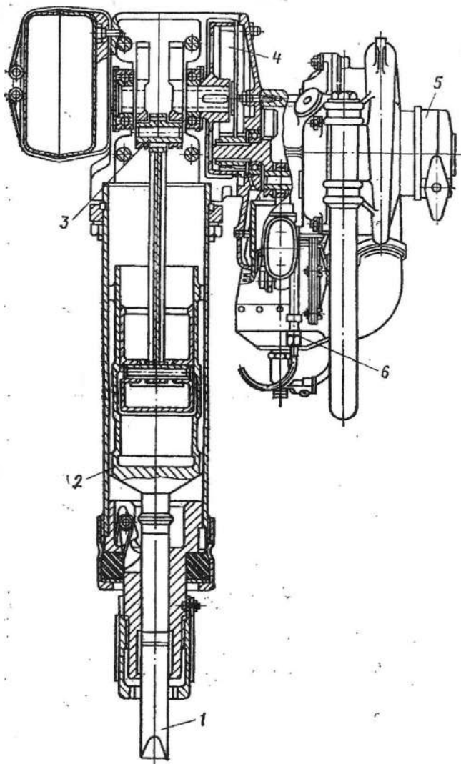
Рис. 15. Мотобетондом.
