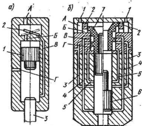
Рис. 9. Схемы воздухораспределения.
