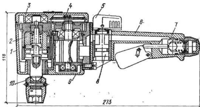
Рис. 8. Пневматический угловой гайковерт ИП-3207А: 1 – корпус; 2 – ударно-импульсный механизм; 3 – верхняя крышка; 4 – пневмодвигатель; 5 – переключатель реверса; 6 – рукоятка; 7 – пусковое устройство; 8 – механизм реверса; 9 – нижняя крышка; 10 – сменная головка.
