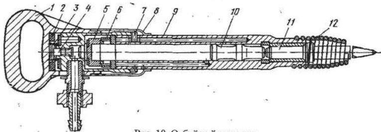
Рис. 10. Отбойный молоток.
