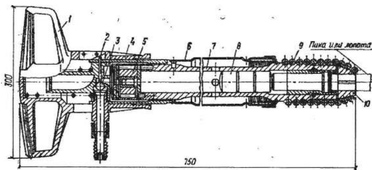
Рис. 12. Бетонолом ИП-4607:
