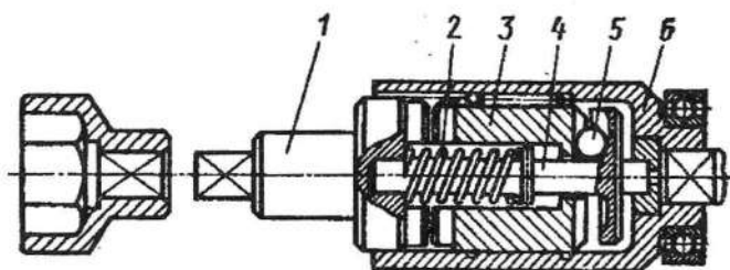
Рис. 5. Ударный механизм пневмогайковерта.
