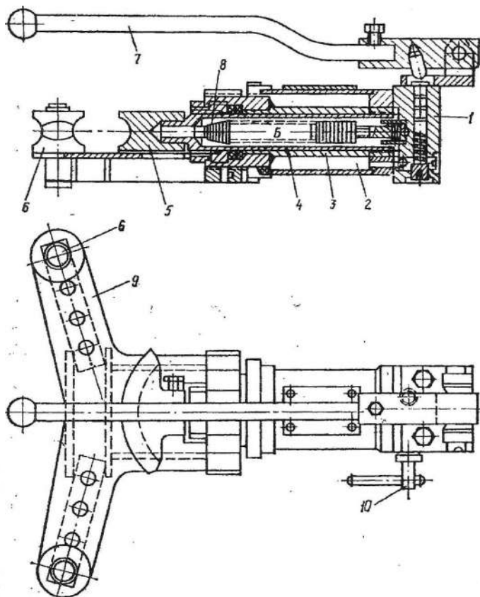
Рис. 16. Гидравлический переносной трубогиб: 1 – насос; 2 – резервуар; 3 – цилиндр; 4 – шток; 5 – головка; 6, 9 – ролики; 7 – рычаг; 8 – пружина; 10 – рукоять спускового клапана.
