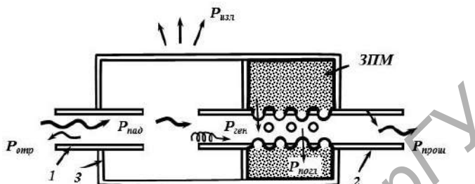
Рис. 1. Распределение потоков звуковой энергии в ГШ: 1 – приемная труба ГШ; 2 – выпускная труба; 3 – корпус ГШ; ЗПМ – звукопоглощающий материал
