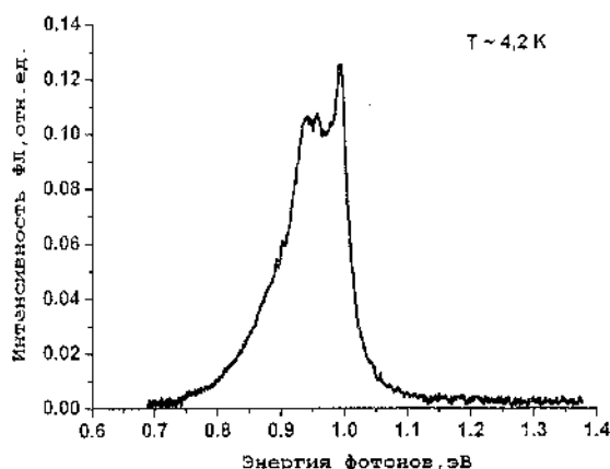
Рисунок 9 — Снятый при 4,2 \text{ К} спектр ФЛ образца Si, имплантированного ионами Sb и In при \text{Sb}^+ \rightarrow \text{Si} : 350 \text{ кэВ} , 3,5 \cdot 10^{16} \text{ см}^{-2} \text{In}^+ \rightarrow \text{Si} : 350 \text{ кэВ} , 3,5 \cdot 10^{16} \text{ см}^{-2} ; T_{\text{импл}} = 500^\circ\text{C} , T_{\text{обр}} = 1100^\circ\text{C} , 30 мин
