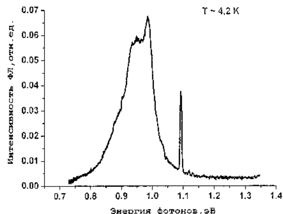
Рисунок 10 — Снятый при 4,2 \text{ К} спектр ФЛ образца \text{SiO}_2(40 \text{ нм})/\text{Si} , имплантированного ионами As и In при \text{As}^+ \rightarrow \text{SiO}_2(40 \text{ нм})/\text{Si} : 170 \text{ кэВ} , 3,2 \cdot 10^{16} \text{ см}^{-2} \text{In}^+ \rightarrow \text{SiO}_2(40 \text{ нм})/\text{Si} : 250 \text{ кэВ} , 2,8 \cdot 10^{16} \text{ см}^{-2} ; T_{\text{импл}} = 500^\circ\text{C} , T_{\text{обр}} = 1050^\circ\text{C} , 3 мин
