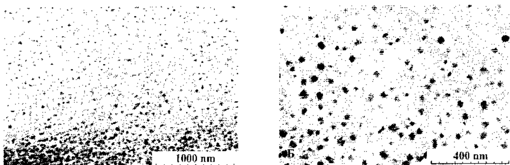
Рисунок 5 — Светлополевые ПЭМ-микрофотографии и гистограммы распределения размеров нанокластеров Sb ( 350\ \text{кэВ} , 3,5 \cdot 10^{16}\ \text{см}^{-2} ) и In ( 350\ \text{кэВ} , 3,5 \cdot 10^{16}\ \text{см}^{-2} ) после отжига при температуре 1\ 100^{\circ}\text{C} в течение 30 мин
