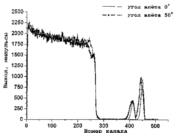
Рисунок 1 — Спектр POP образца кремния, имплантированного ионами \text{In}^+ (350 кэВ, 3,5 \cdot 10^{16} \text{ см}^{-2} ) \text{Sb}^+ (350 кэВ, 3,5 \cdot 10^{16} \text{ см}^{-2} )
