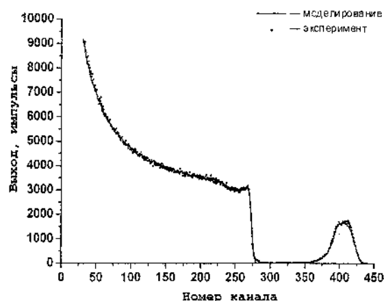
Рисунок 2 — Спектр POP образца кремния, имплантированного ионами \text{In}^+ (250 кэВ, 2,8 \cdot 10^{16} \text{ см}^{-2} ) \text{As}^+ (170 кэВ, 3,2 \cdot 10^{16} \text{ см}^{-2} ), для двух различных влётов ионов гелия
