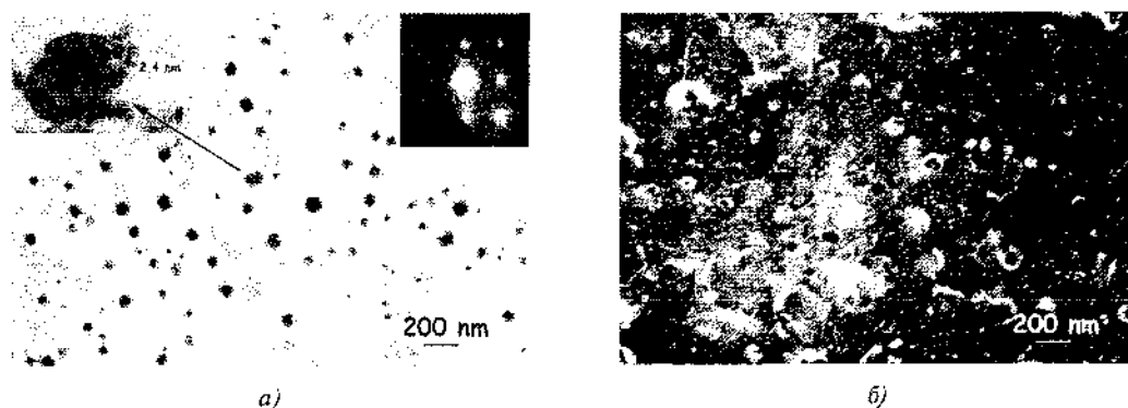
Рисунок 6 — Светлополевая (а) и тёмнополевая (б) ПЭМ-микрофотографии после имплантации ионов As ( 170\ \text{кэВ} , 3,2 \cdot 10^{16}\ \text{см}^{-2} ) и In ( 250\ \text{кэВ} , 2,8 \cdot 10^{16}\ \text{см}^{-2} ) и последующего отжига при температуре 1\ 050^{\circ}\text{C} в течение 30 мин
