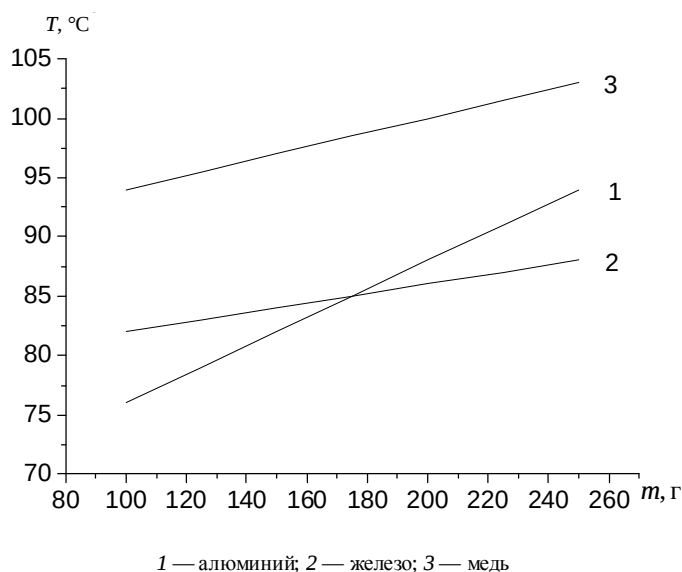
Рисунок 4 — Зависимость конечной температуры T , °C, прессуемой детали от её массы m
