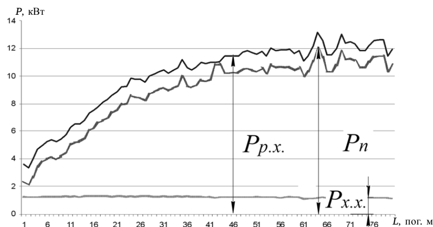
Рисунок 3 — Шлифование древесины сосны при скорости резания 18 м / с, скорости подачи 8 м / мин, припуске на обработку 0,4 мм, зернистости Р80
