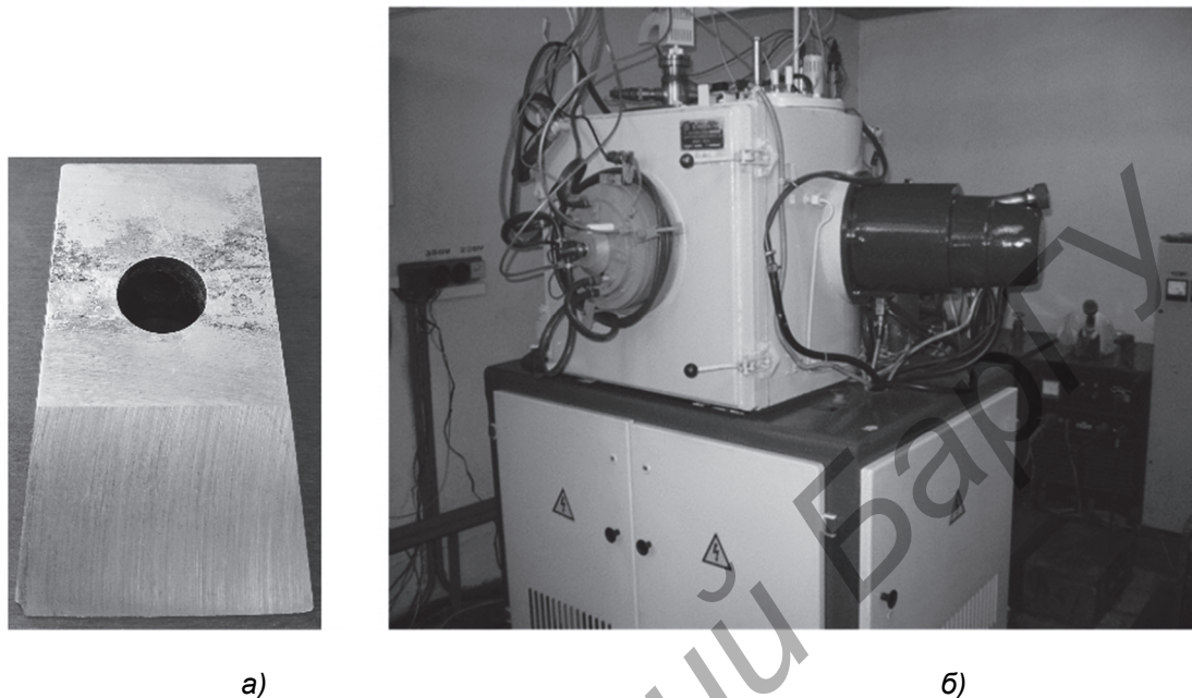
Рисунок 1. — Вид рубительного ножа (а) и оборудования ННВ 6,6-И1 с двухлучевым распылительным ионным источником ИРЛУ-2 и катодным узлом ARC (б)
