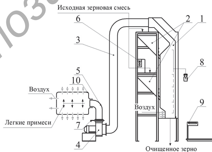
1 — лабораторный макет пневматического канала окончательной аспирации МУЗ-16; 2 — бункера для исходной зерновой смеси; 3, 5 — воздуховод; 4 — вентилятор; 6 — магнитный пускатель двигателя вентилятора; 7 — заслонка; 8 — термоанометр; 9 — весы; 10 — фильтровальная перегородка
